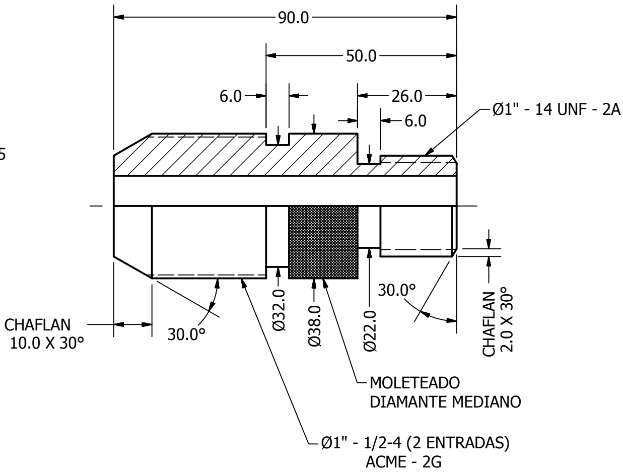
MEDIA SECCIÓN C-C
